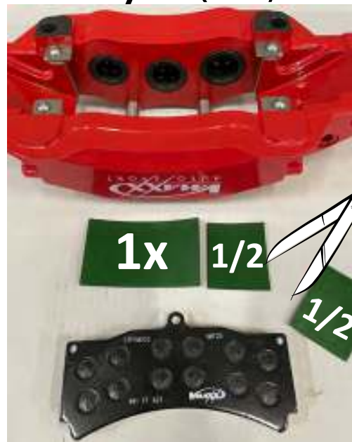
24C VM 05 / 06 (Ø 355/365mm BBK)
